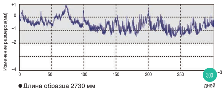
Изменение длины 16 мм сайдинга других производителей
