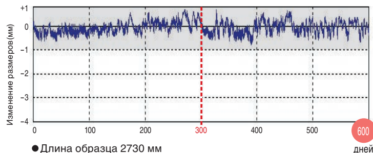
Изменение длины материала серии «Серадир»
